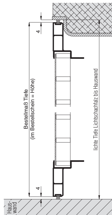
Vertikalschnitt Tiefe (Seitenansicht)
