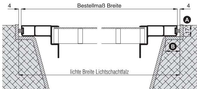
Vertikalschnitt Breite (Vorderansicht)
